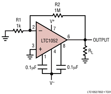
LTC1052/7652 • TC01
