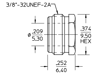
CLAMP NUT
