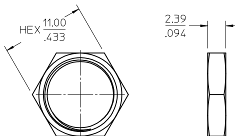
JAM NUT
