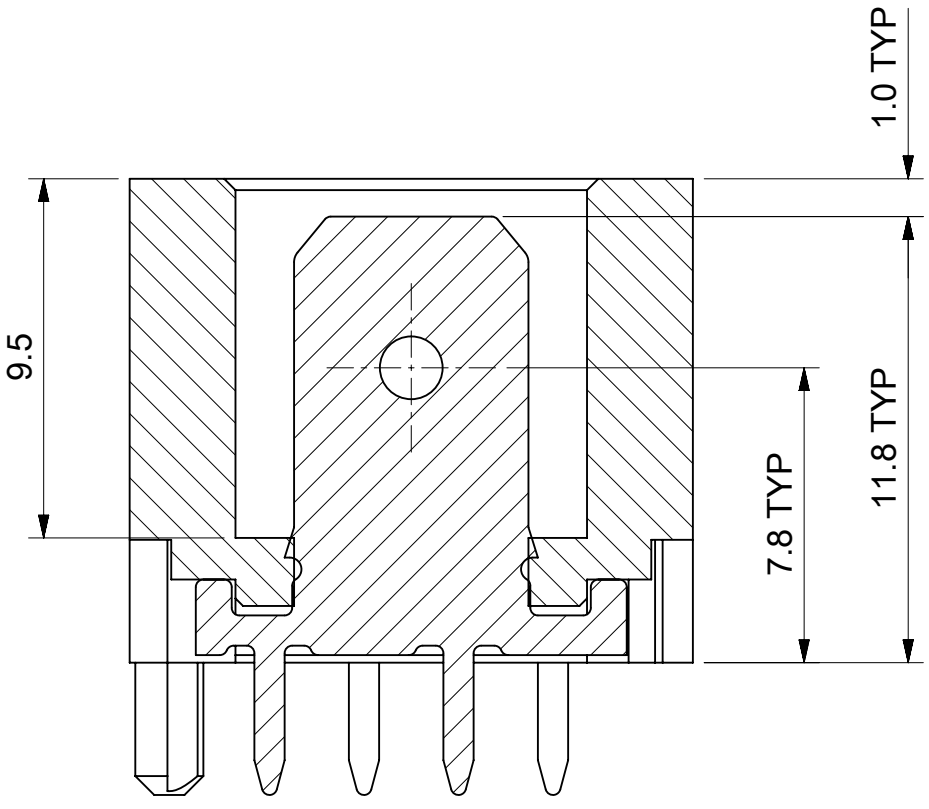
SECTION A-A
