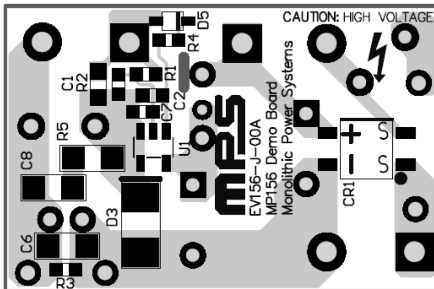
Figure 3 — Bottom Layer
