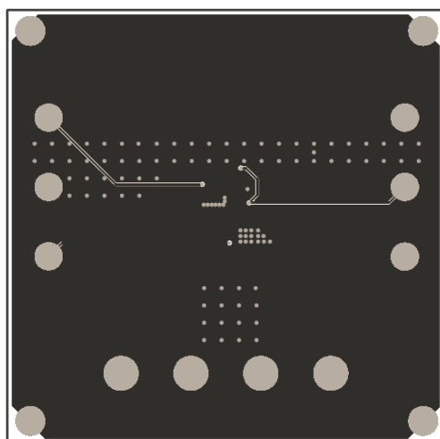
Figure 4—Bottom Layer
