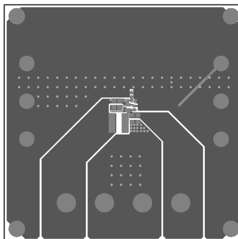
Figure 3—Top Layer
