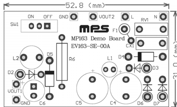
Figure 2—Top Layer
