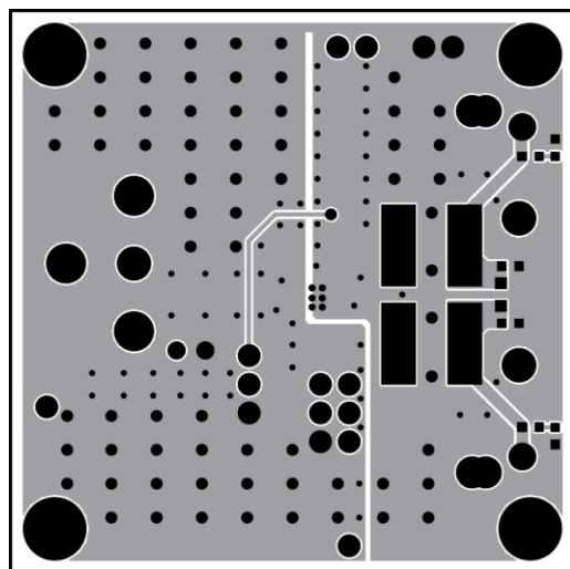
Figure 3—Bottom Layer
