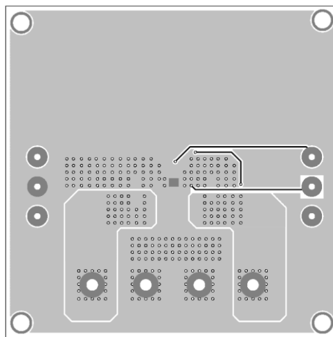
Figure 2—Bottom Layer
