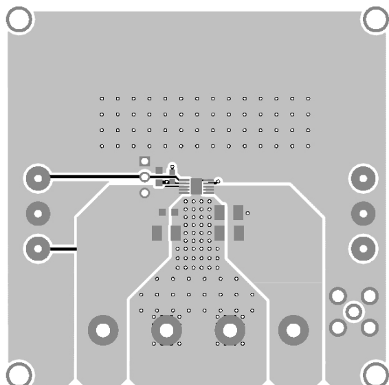
Figure 1—Top Layer
