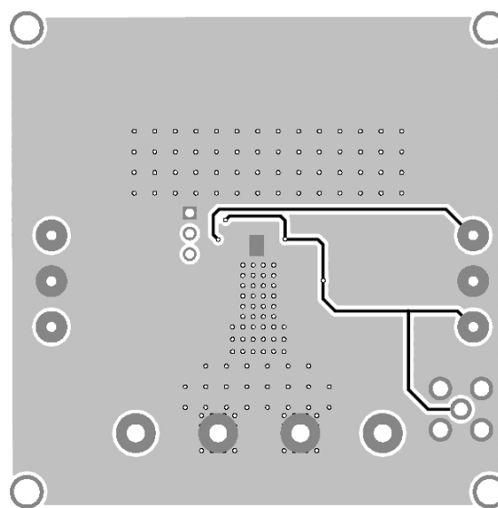
Figure 2—Bottom Layer
