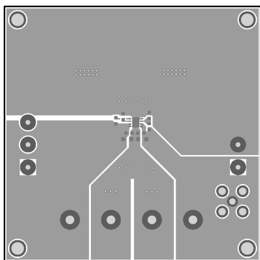
Figure 1—Top Layer
