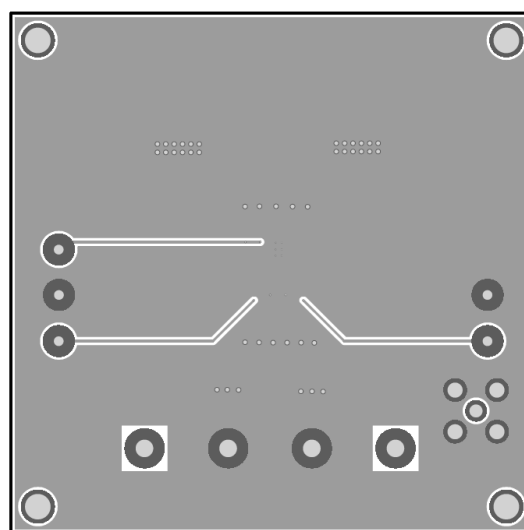
Figure 2—Bottom Layer
