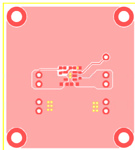
Figure 3—Top Layer
