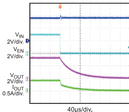
Enable Off
