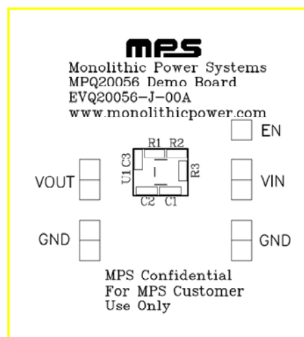
Figure 2—Top Silk Layer
