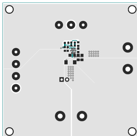
Figure 2—Top Layer
