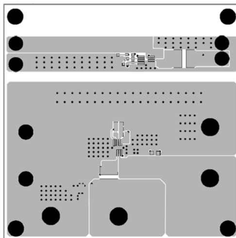
Figure 2—Top Layer
