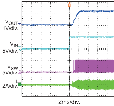
Enable On
