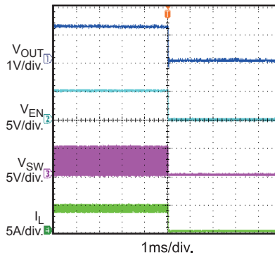
Enable Shutdown
