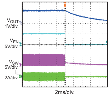
Enable Shutdown
