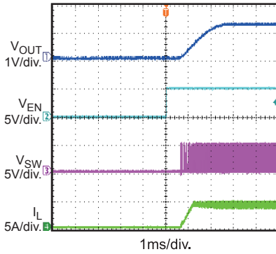
Enable On
