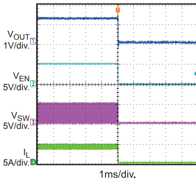
Enable Shutdown
