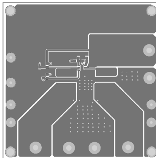
Figure 2—Top Layer
