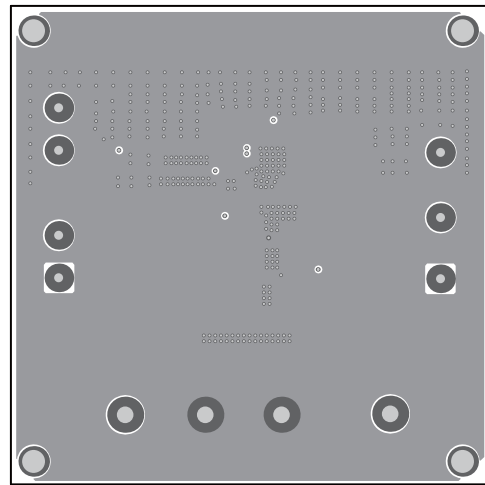
Figure 4—IN2 Layer
