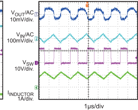
Input/Output Ripple
