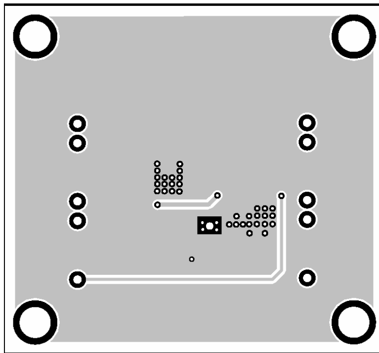
Figure 2—Bottom Layer
