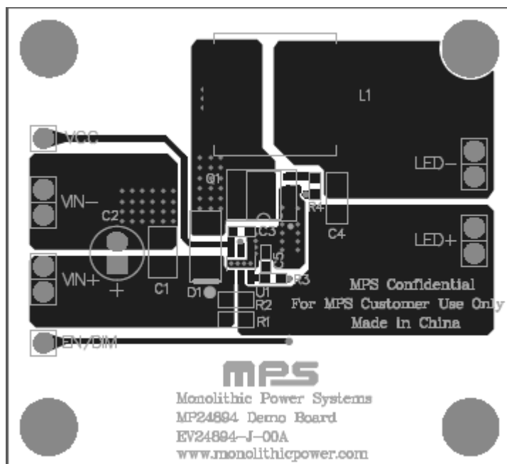
Figure 1—Top Layer
