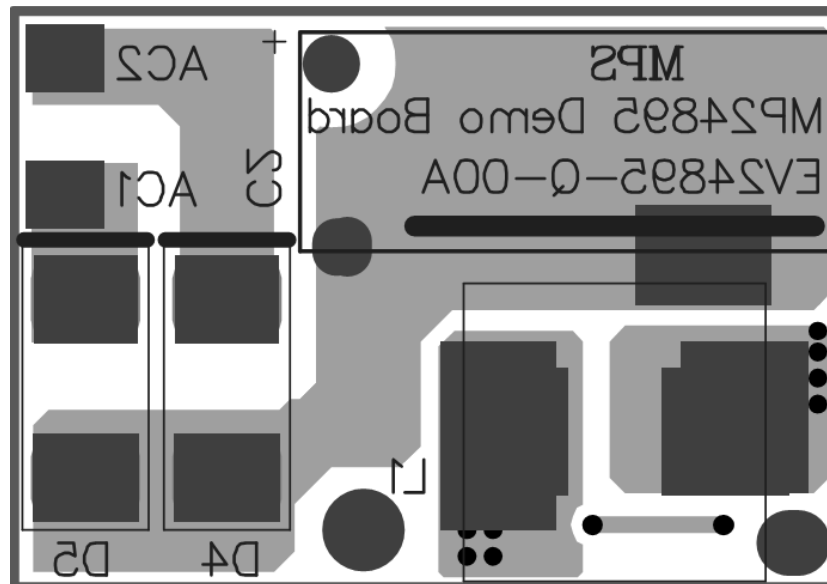
Figure 2—Bottom Layer
