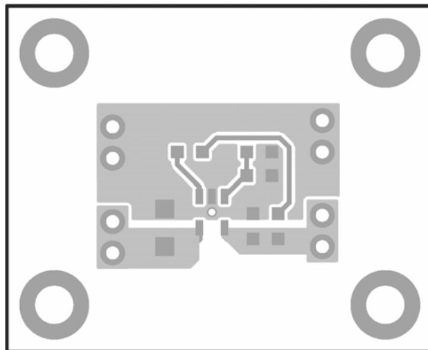
Figure 2—Top Layer
