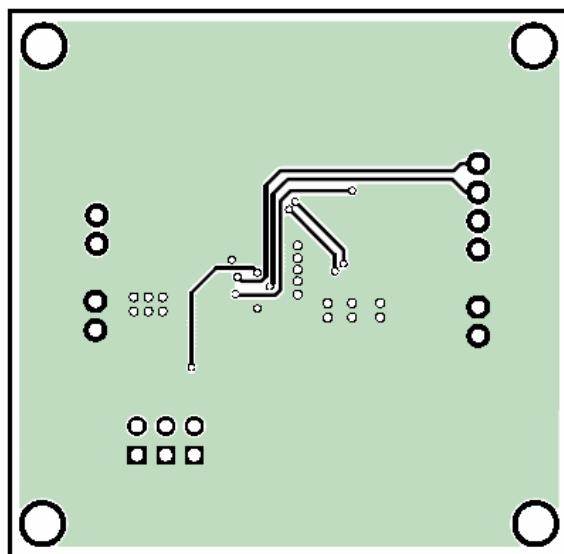
Figure 3—Bottom Layer
