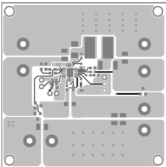
Figure 1—Top Layer
