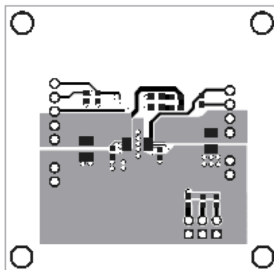
Figure 2—Top Layer
