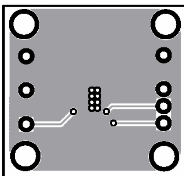
Figure 3—Bottom Layer
