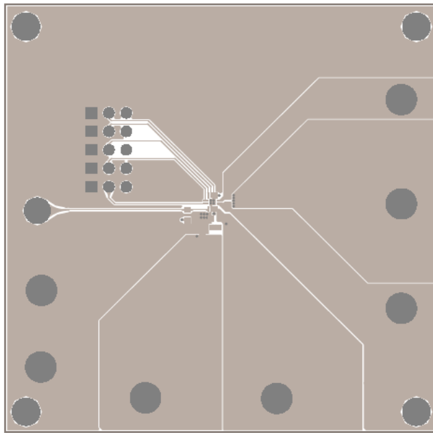
Figure 5—Top Layer
