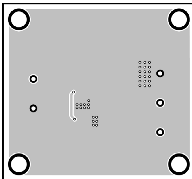
Figure 2—Bottom Layer
