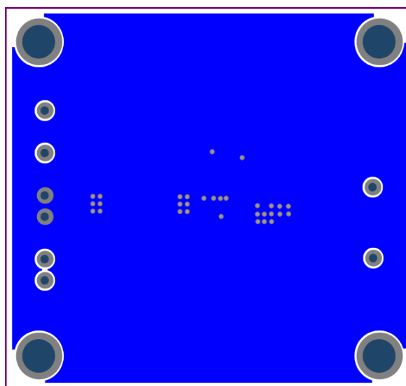
Figure 2—Bottom Layer
