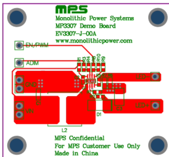
Figure 1—Top Layer
