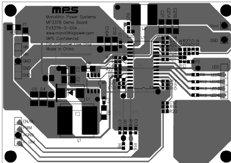
Figure 1—Top Layer
