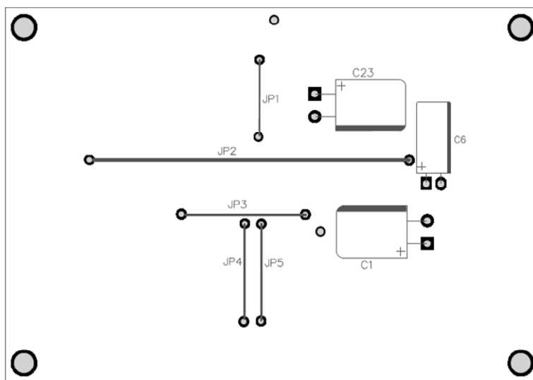
Figure 2—Bottom Layer
