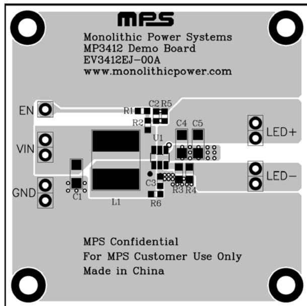
Figure 1—Top Layer
