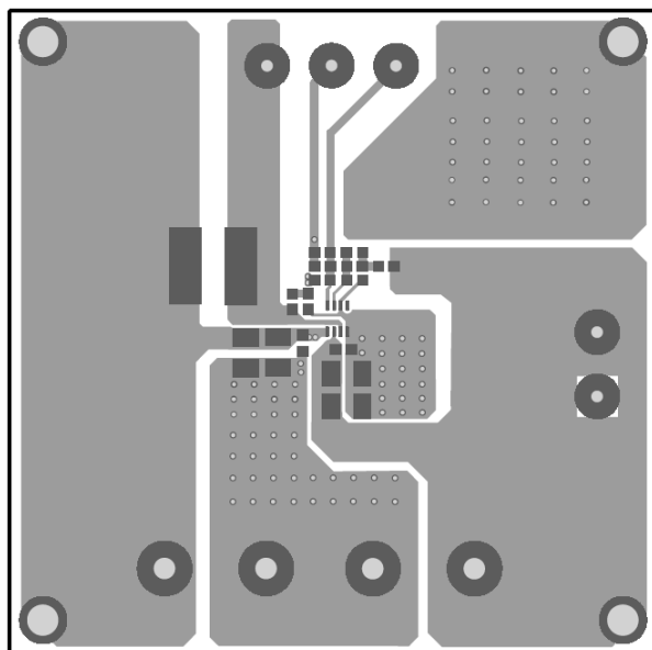
Figure 1—Top Layer
