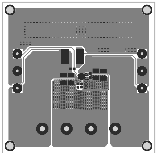
Figure 2—Top Layer
