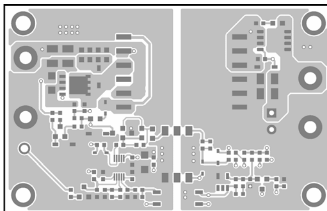
Figure 2—Top Layer
