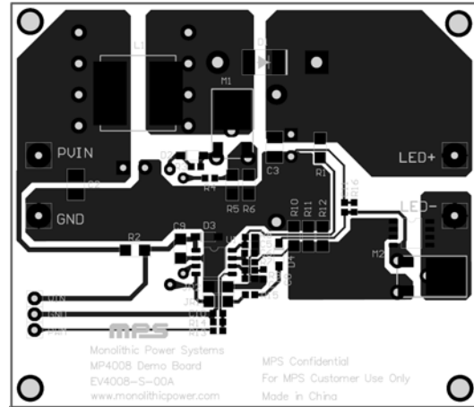
Figure 2—Top Layer
