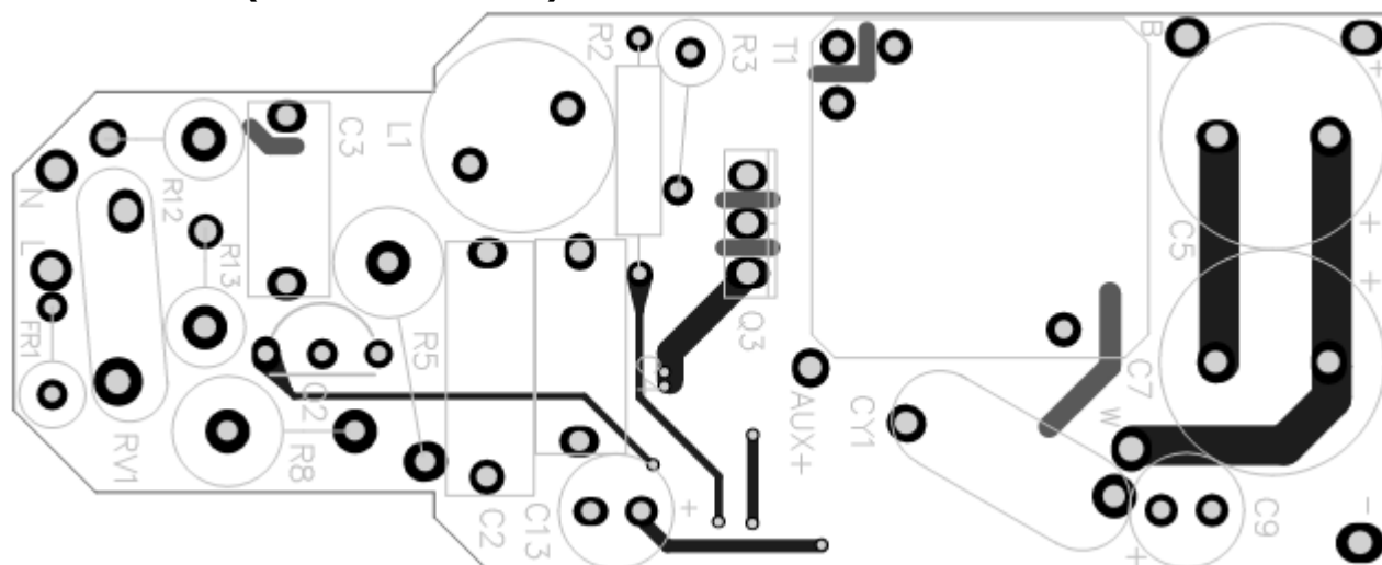
Figure 2—Top Layer
