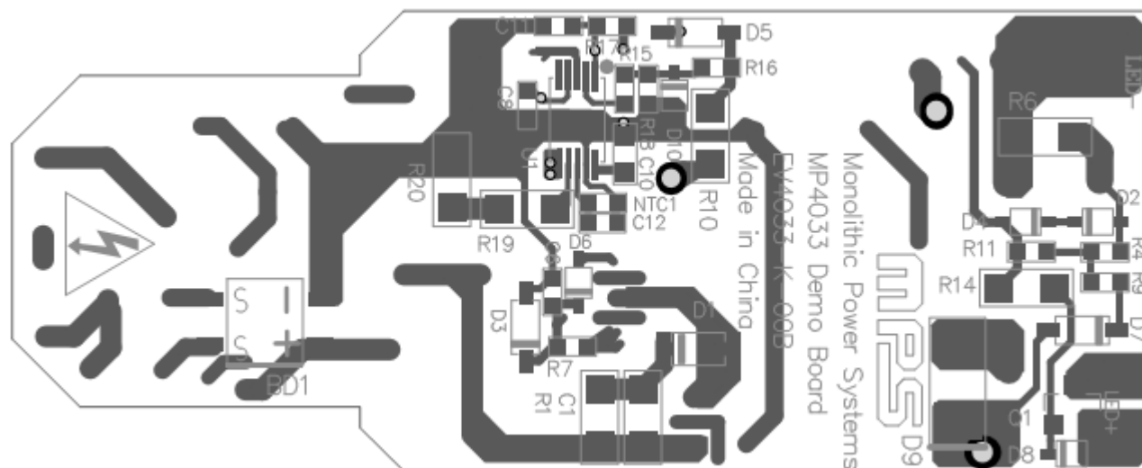
Figure 3—Bottom Layer
