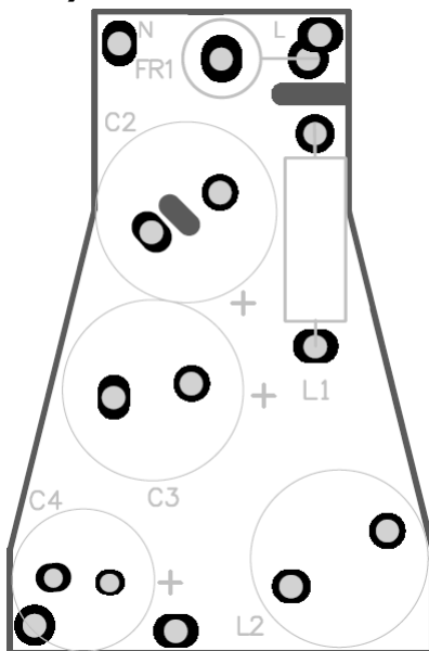
Figure 2—Top Layer
