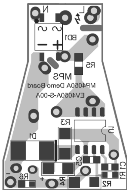
Figure 3—Bottom Layer
