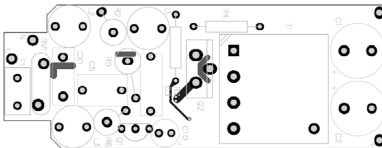
Figure 2—Top Layer
