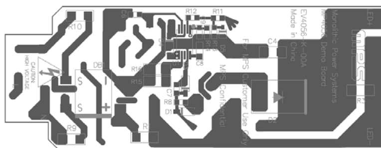
Figure 3—Bottom Layer
