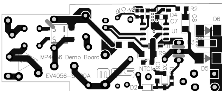
Figure 3—Bottom Layer
