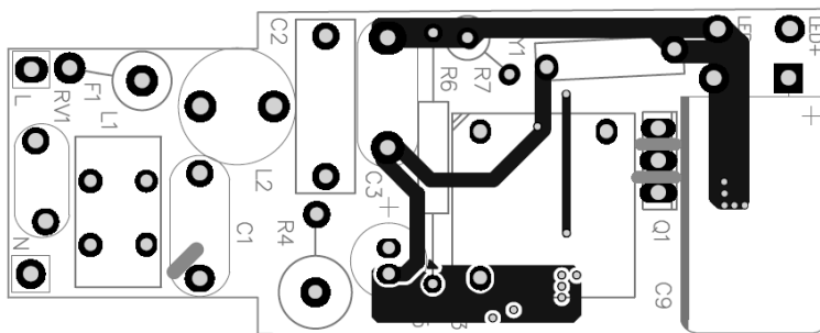
Figure 2—Top Layer
