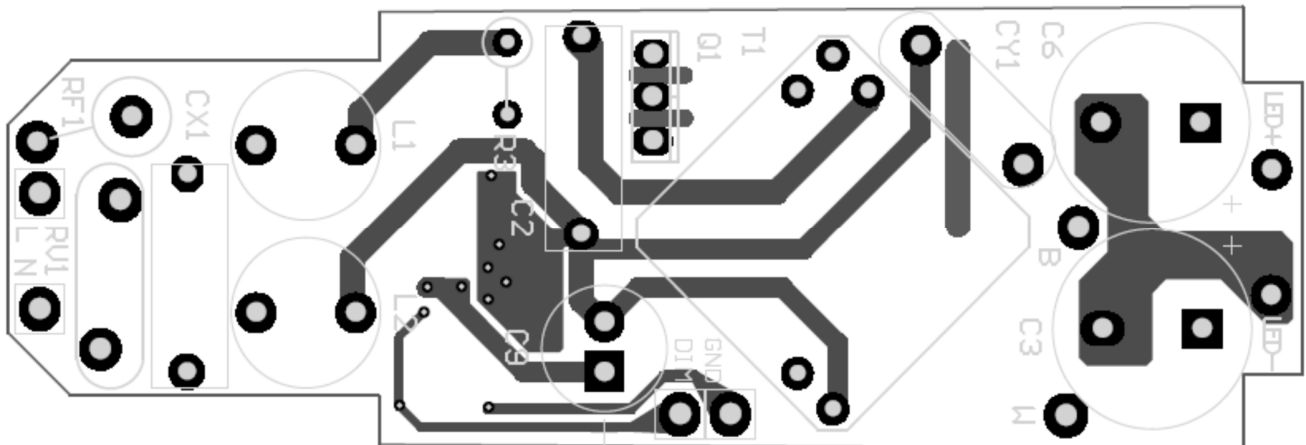
Top layer
