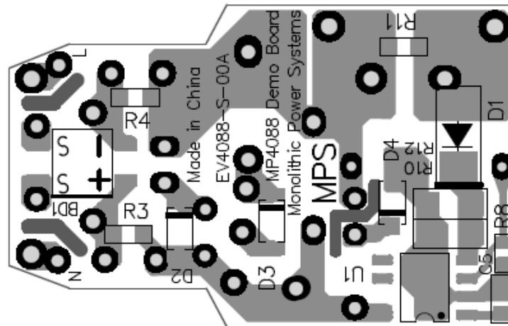
Figure 3—Bottom Layer
