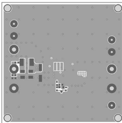
Figure5 – Bottom Layer
