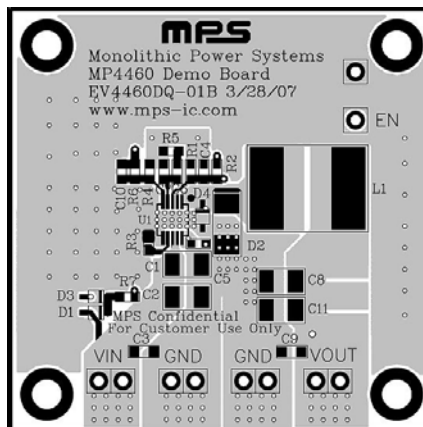
Figure 2—Top Layer
