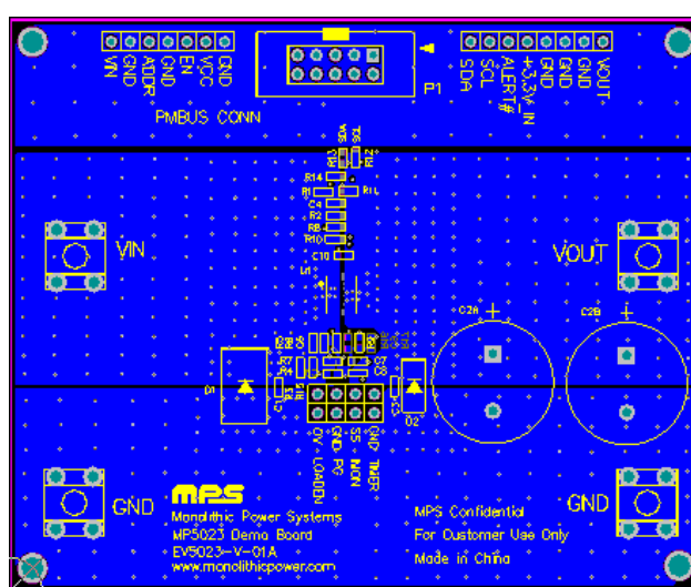
Figure 4—Bottom Layer
