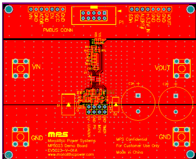
Figure 1—Top Layer
