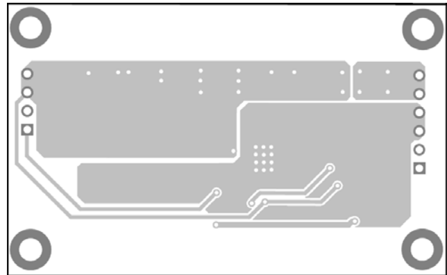
Bottom Layer
