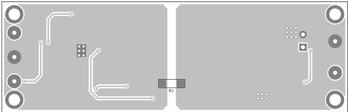
Figure 2—Bottom Layer
