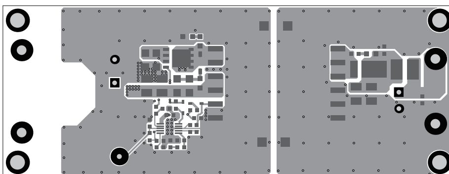
Figure 2—Top Layer
