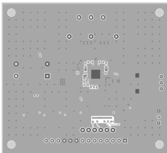
Figure 5—Bottom Layer
