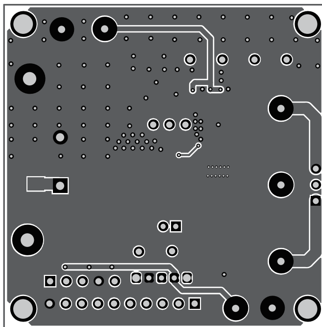
Figure 3—Bottom Layer
