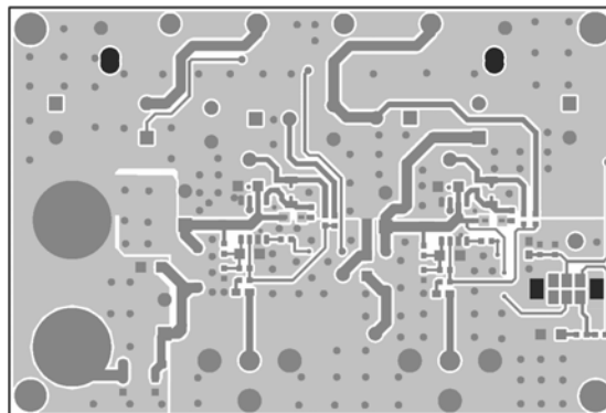
Figure 2—Top Layer
