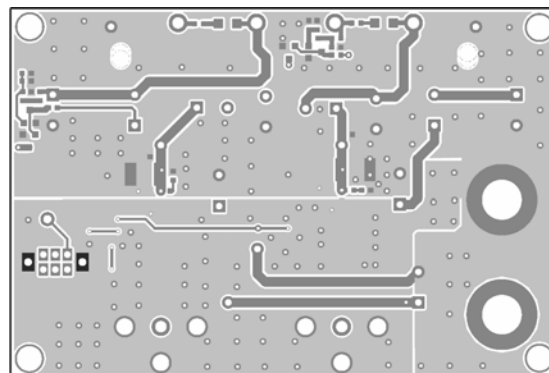
Figure 4—Bottom Layer
